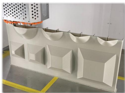
3D プリンティングによる樹脂製型枠の造形
